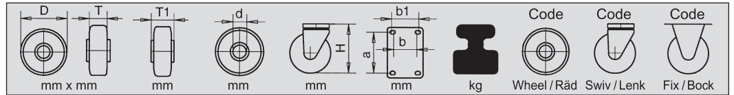
Standard phenolic resin, plain bore, with zinc plated / Standard phenolharz-Gleitlager mit verzinkter Gabel
